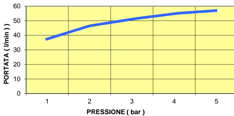
T140 PORTATA FLOW
