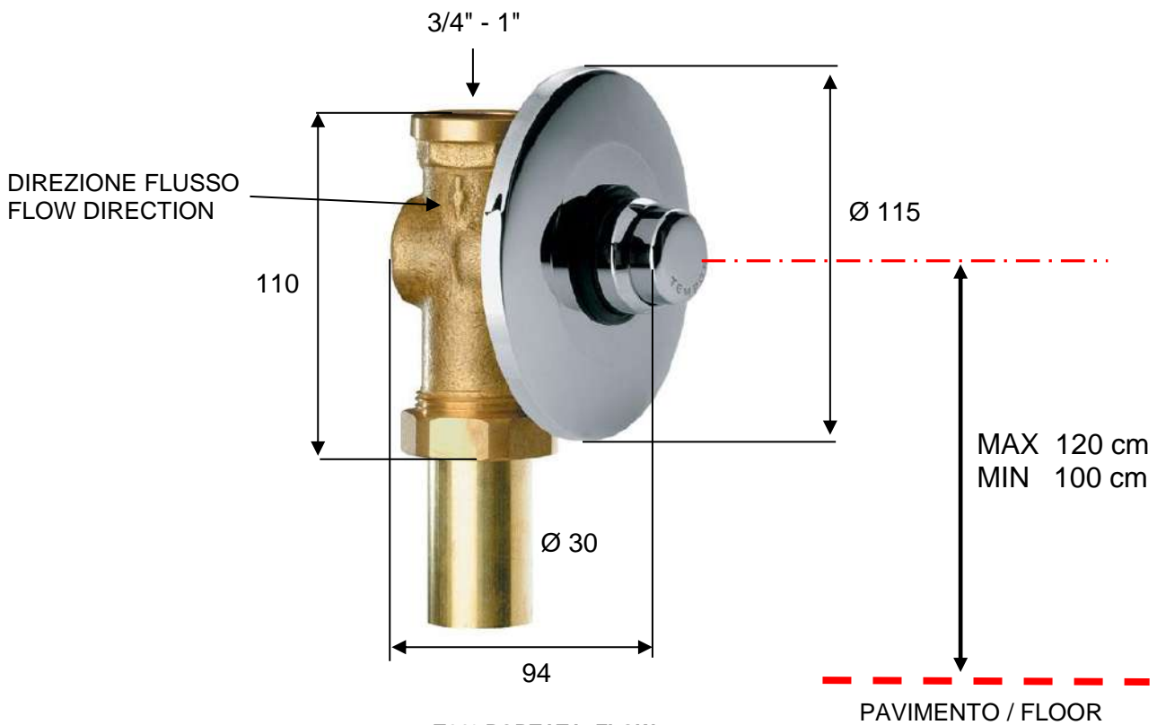
T140 PORTATA FLOW
